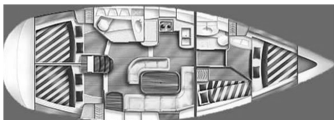
- Gib sea 43(Luna V) Layout
