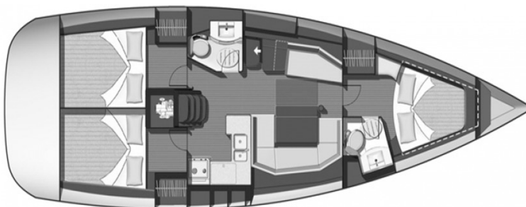
- Sun Odyssey 42 i(Minidora) Layout
